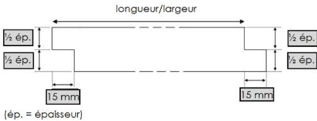
Fig. 1 – feuillureComposants auxiliaires
